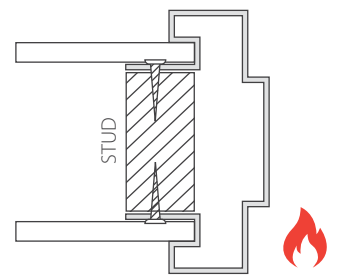
NEW GEN FRAME
