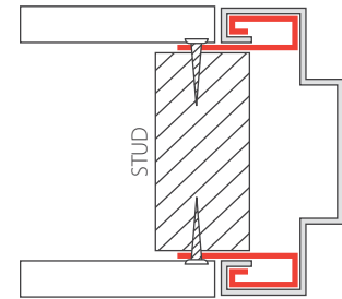
STUD CLIPS (LOOSE)
